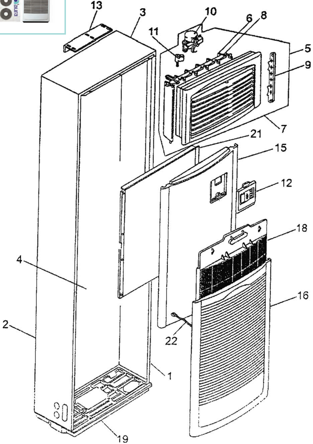
Şekil 81A - İç Ünite
