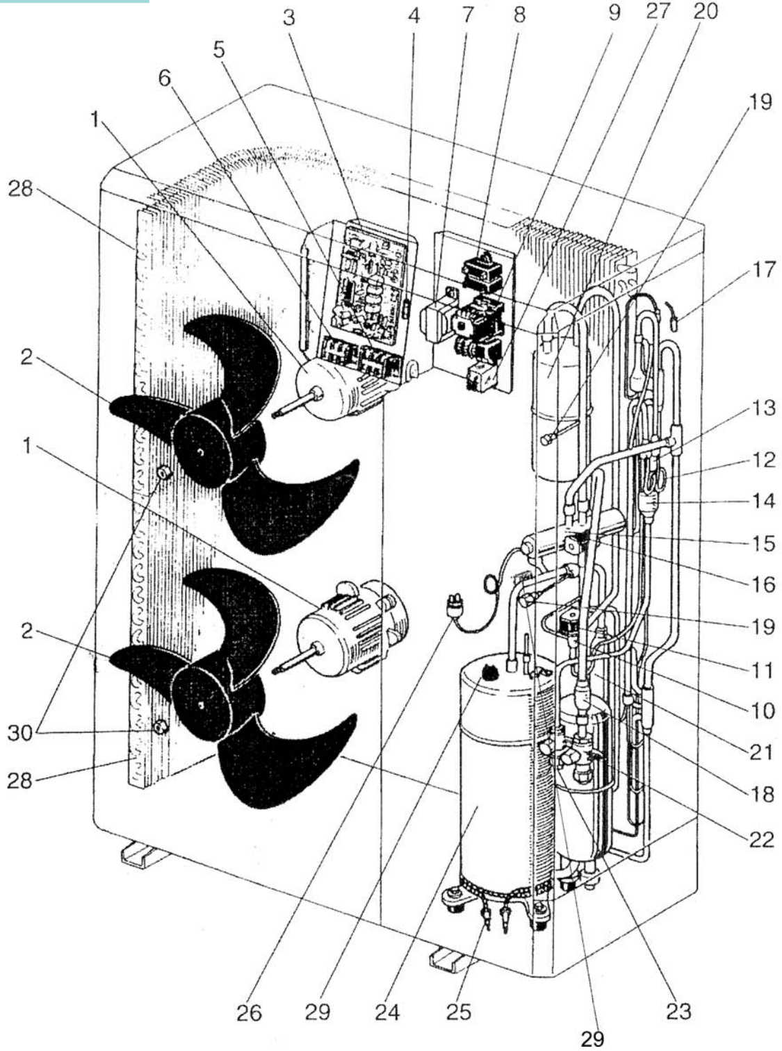
Şekil 81B - Dış Ünite
