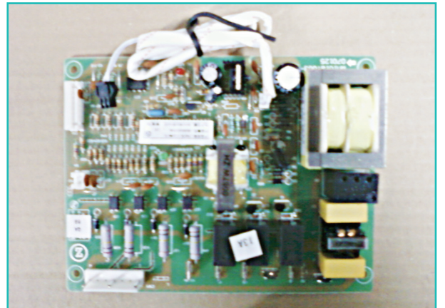
42000 BTU Dış Ünite Kartı
