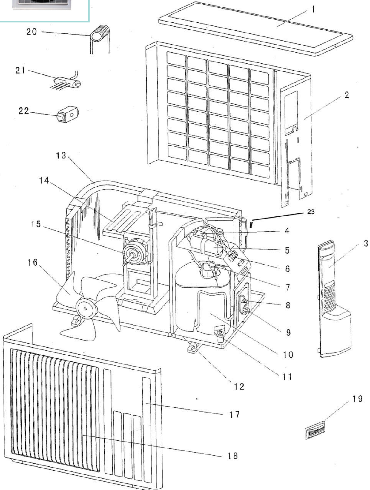
Şekil 77B - Dış Ünite
