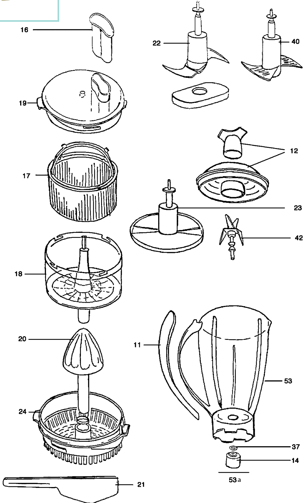
Şekil 55B - Hazne Grubu
