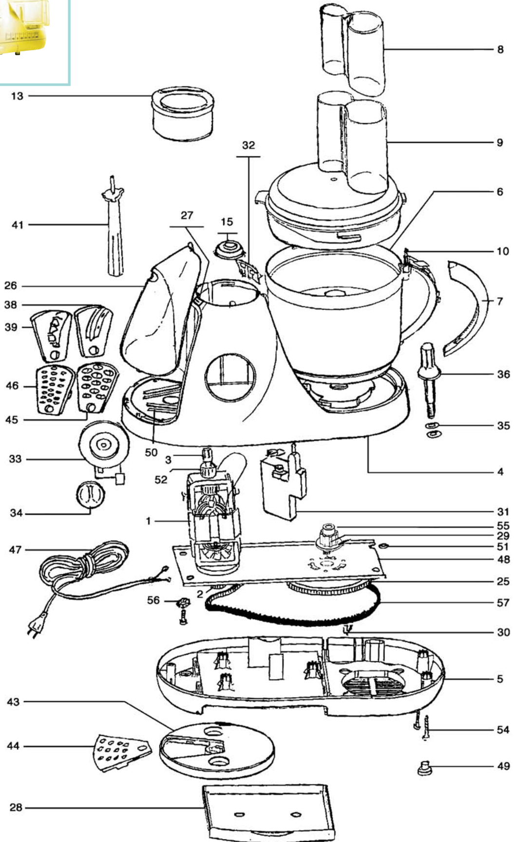
Şekil 55A - G vde Grubu
