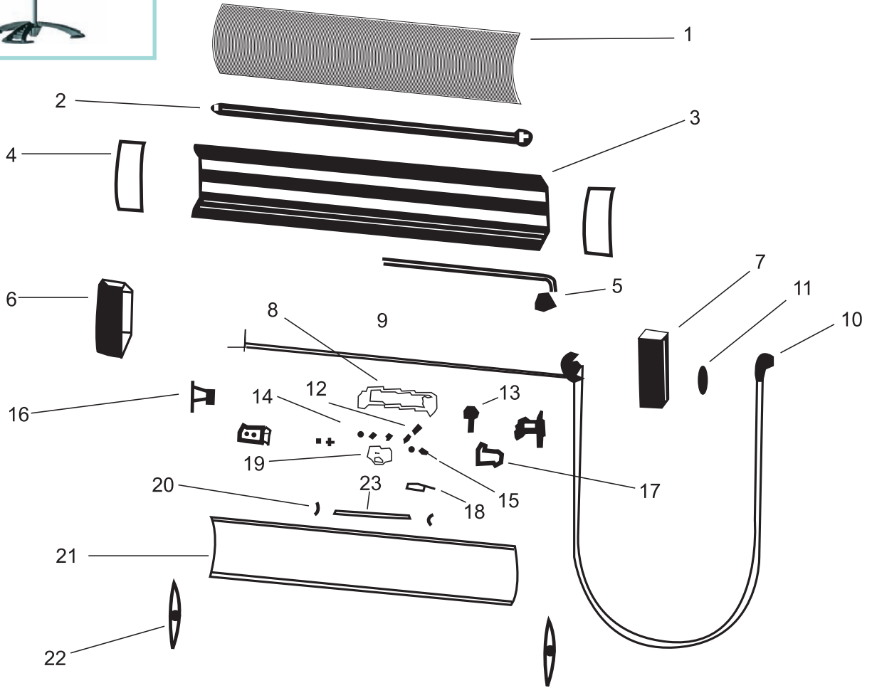
Şekil 71A - Isıtıcı Grubu
