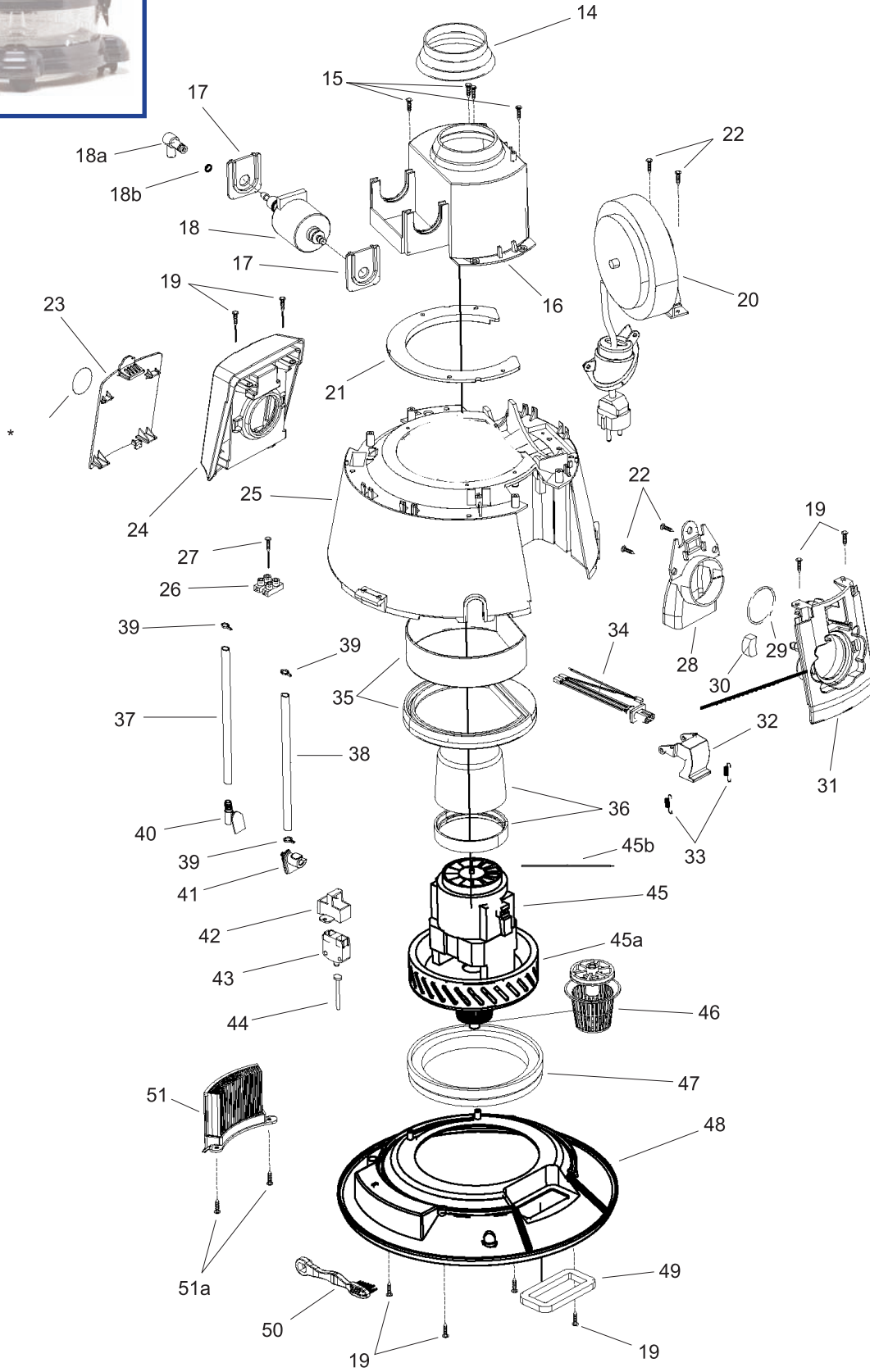
Şekil 2B - Gövde Grubu
