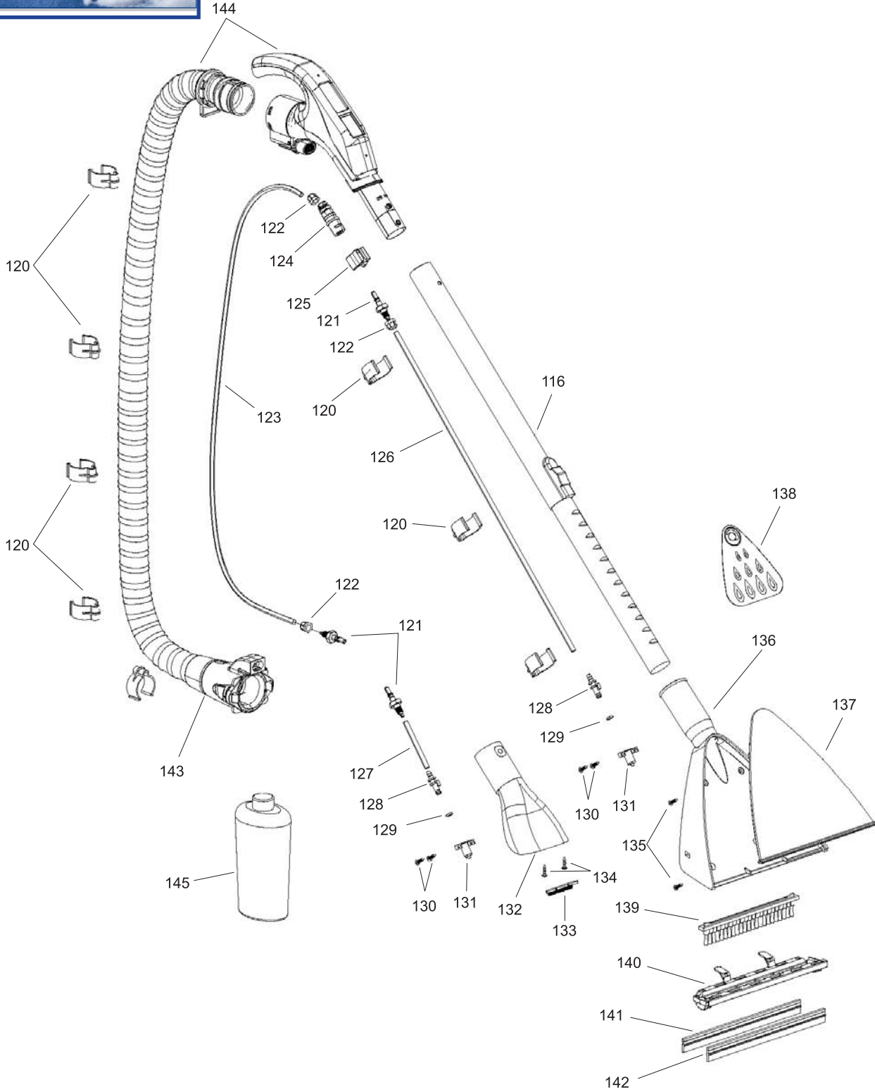
Şekil 2F - Yıkama Grubu
