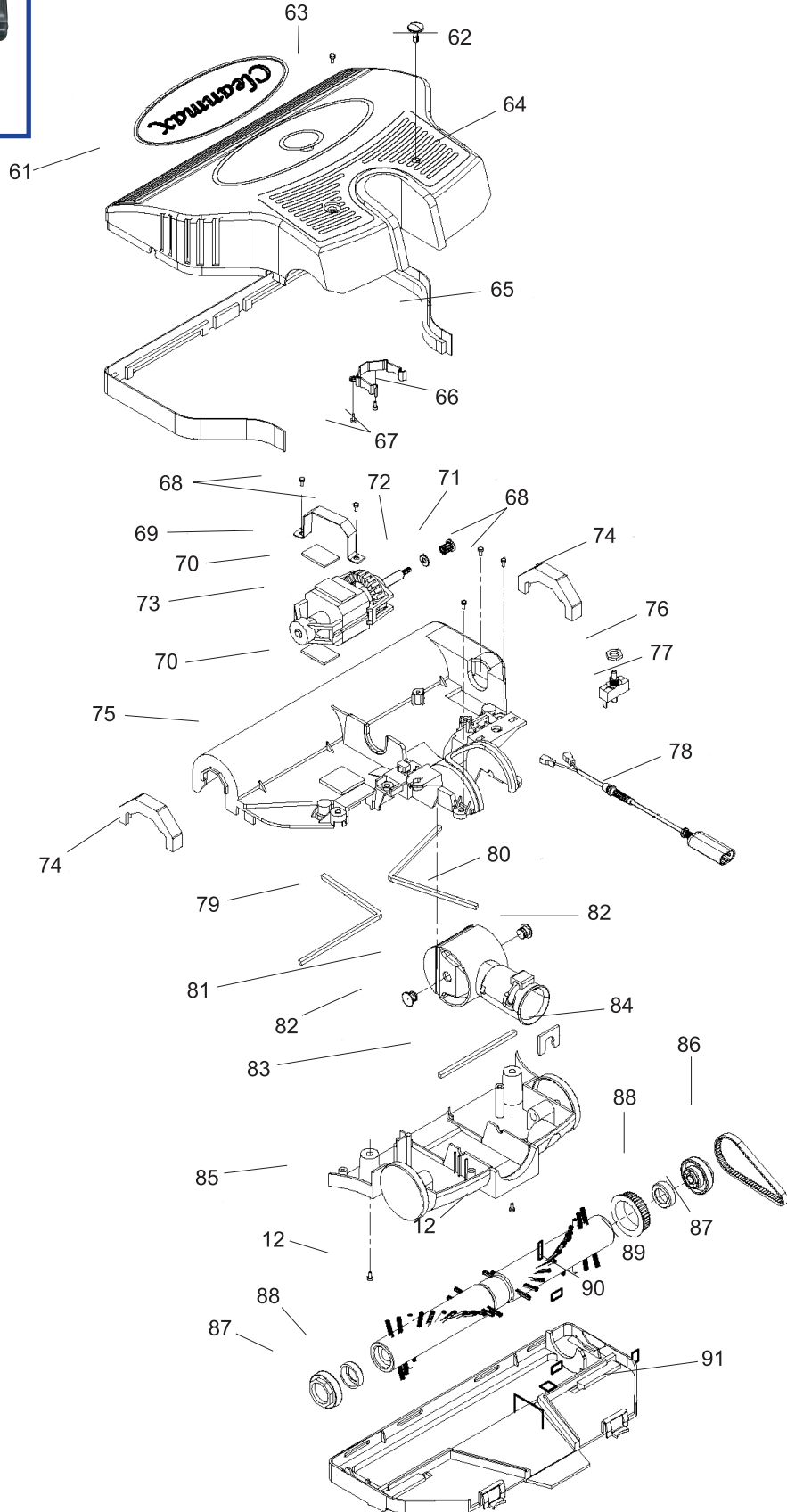
Şekil 2D - Derin Dövücü Grubu
