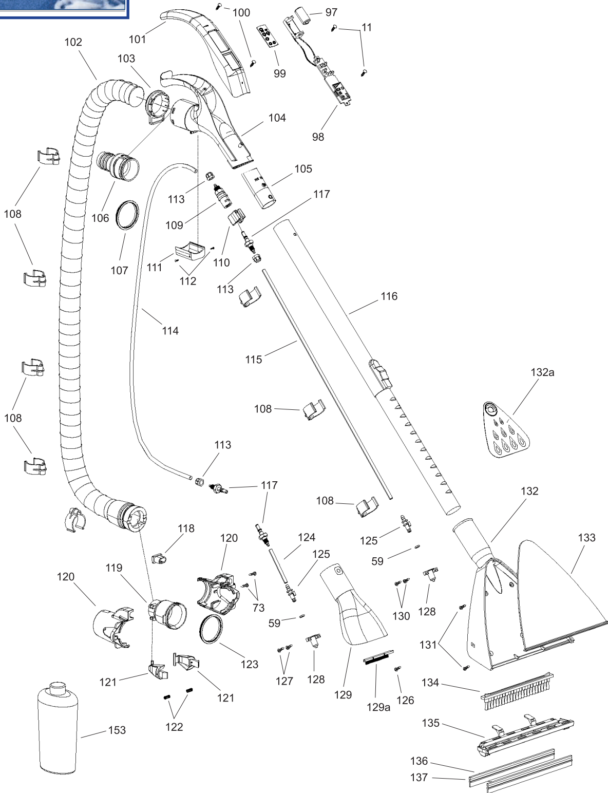
Şekil 1E - Yıkama Grubu
