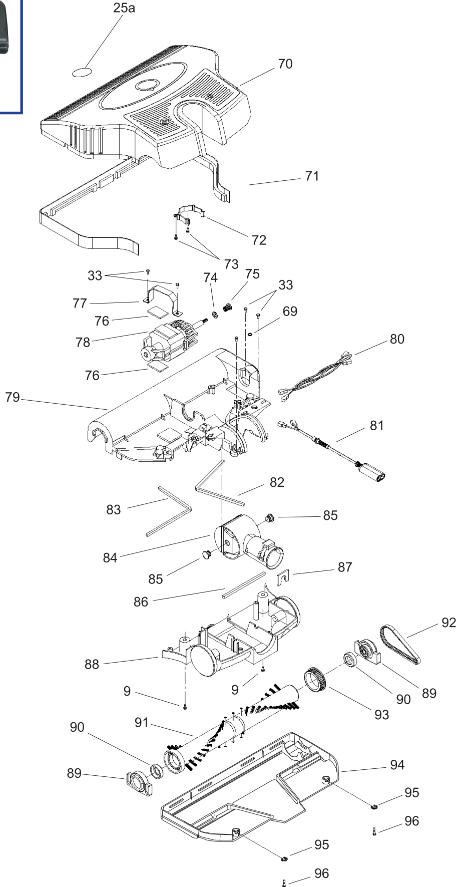
Şekil 1I - Derin Dövücü Grubu (Eski Model)
