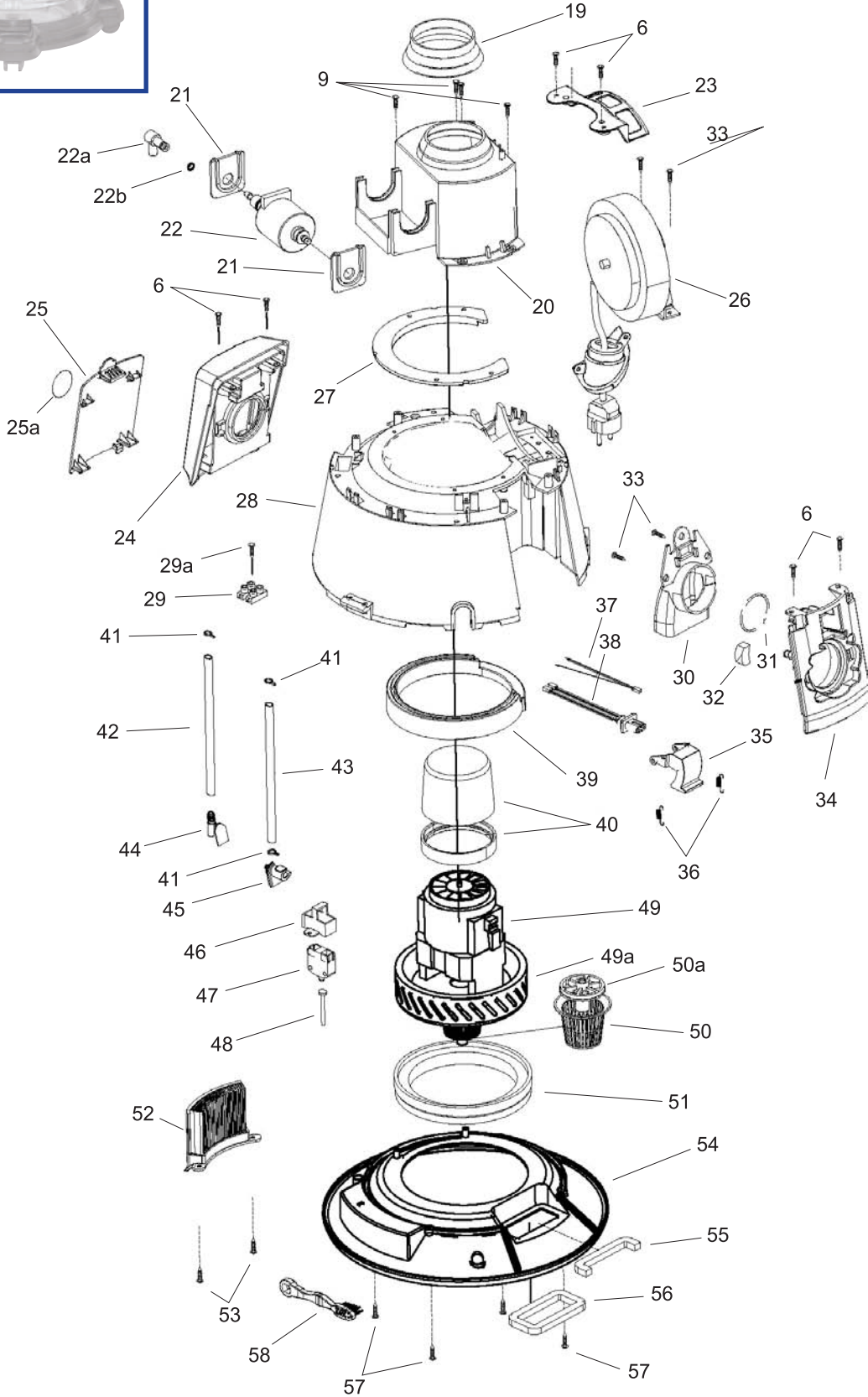
Şekil 1B - Gövde Grubu
