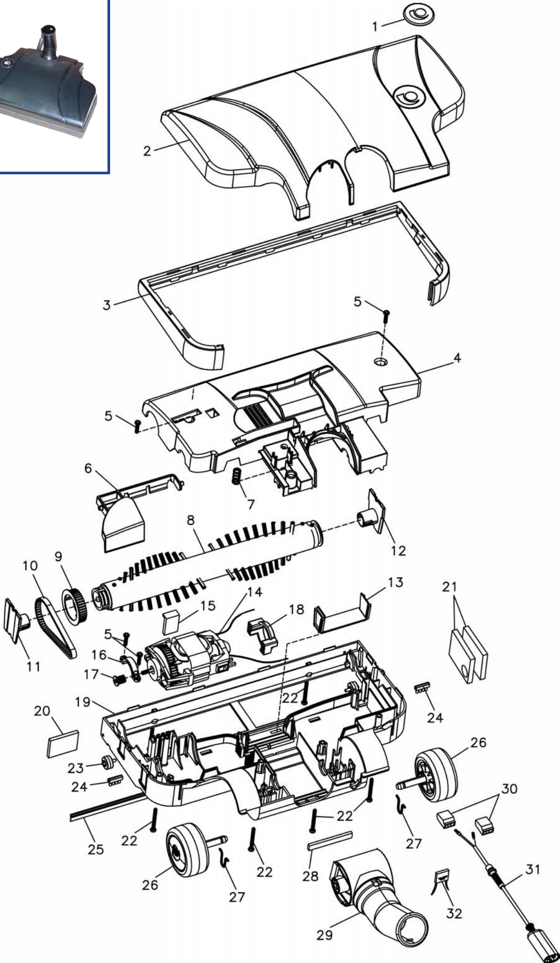
Şekil 1F - Derin Dövücü Grubu (v2007)
