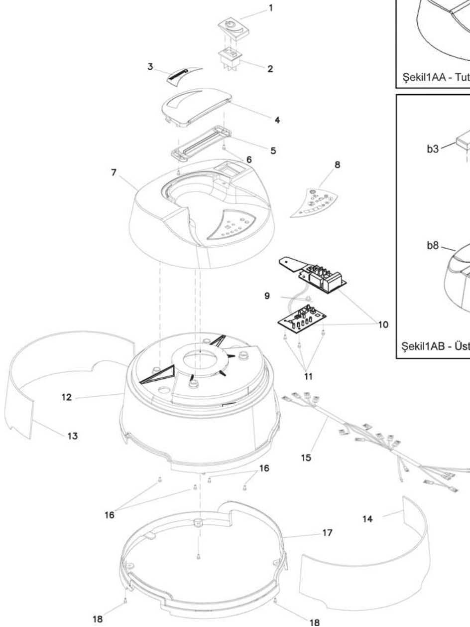
Şekil 1A - Üst Gövde Grubu
