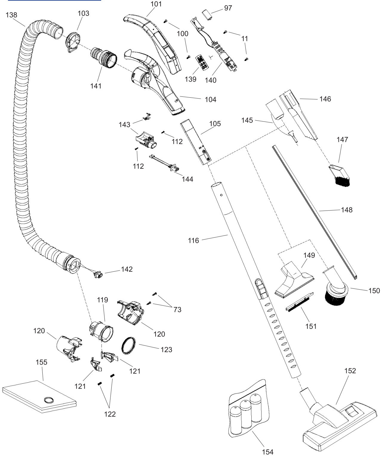
Şekil 1D - Süpürme Grubu
