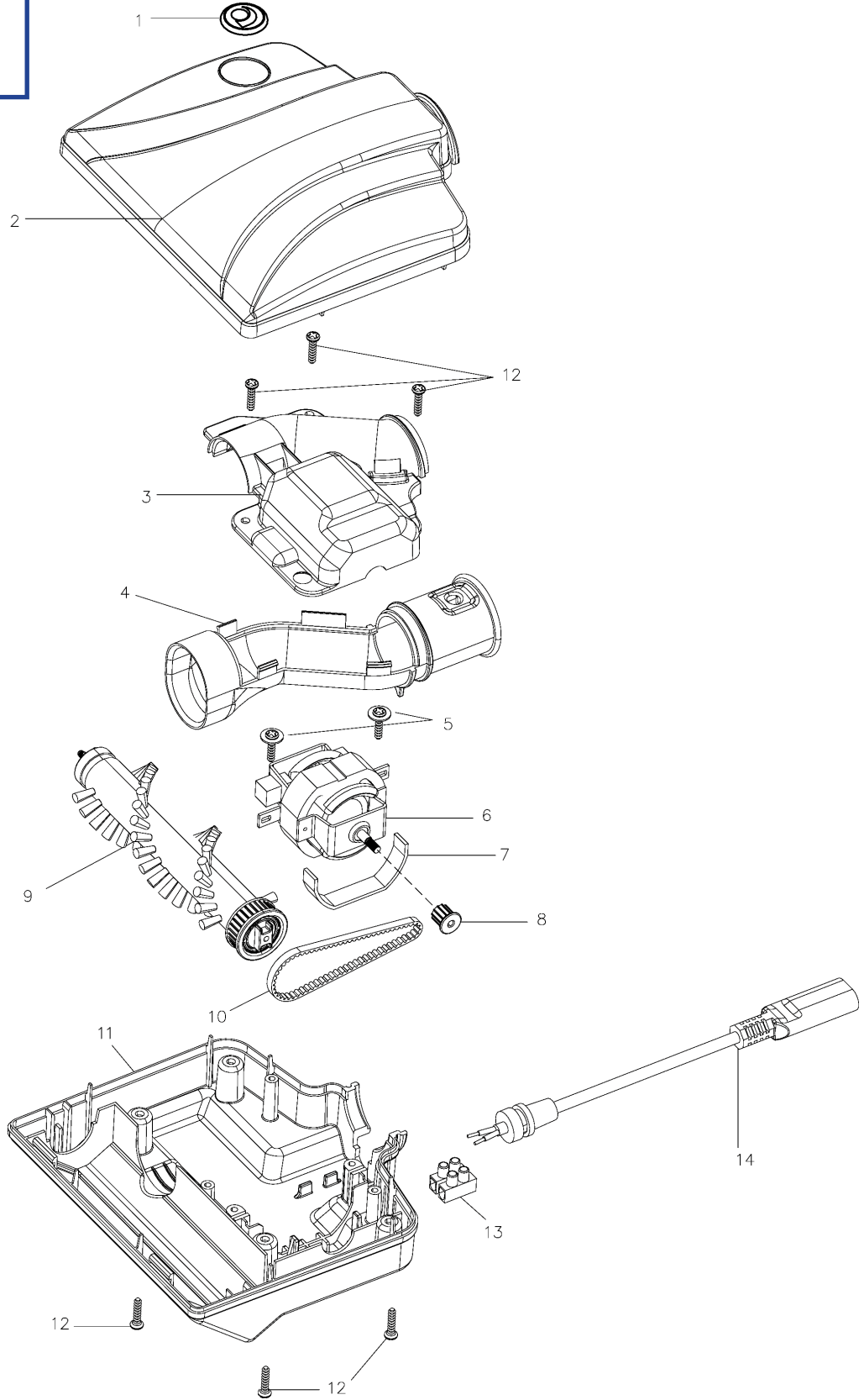
Şekil 1G - Küçük Dövecü Grubu
