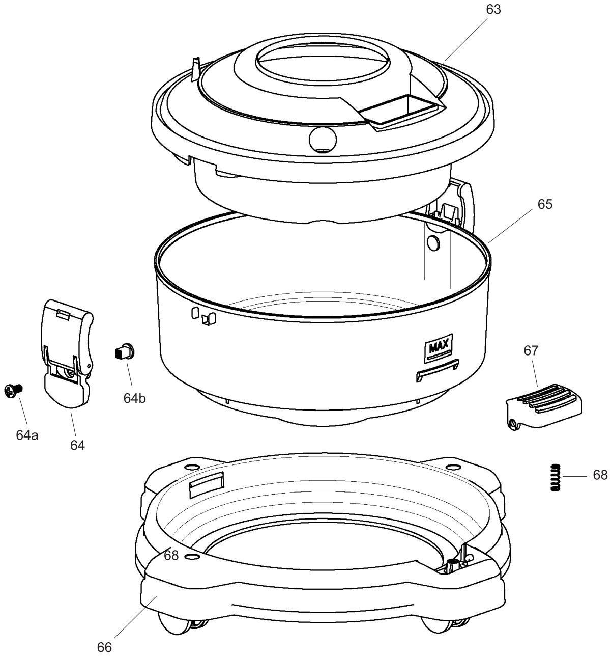
Şekil 1C - Yıkama Hazne Grubu
