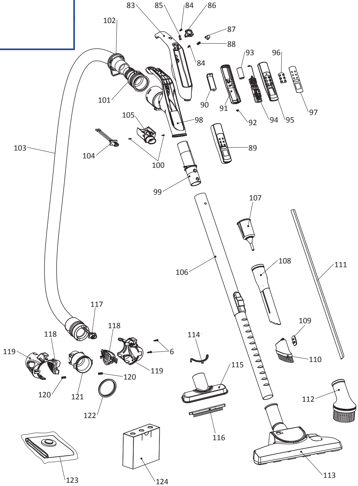
Şekil 1D - Süpürme Grubu
