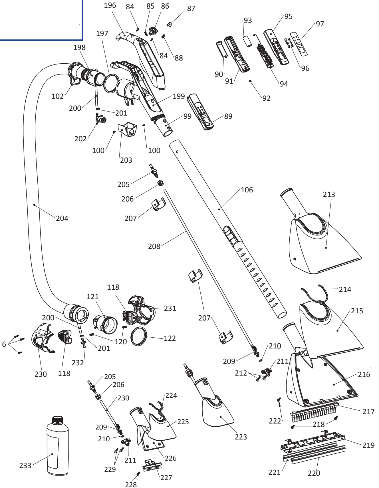
Şekil 1H - Yıkama Grubu
