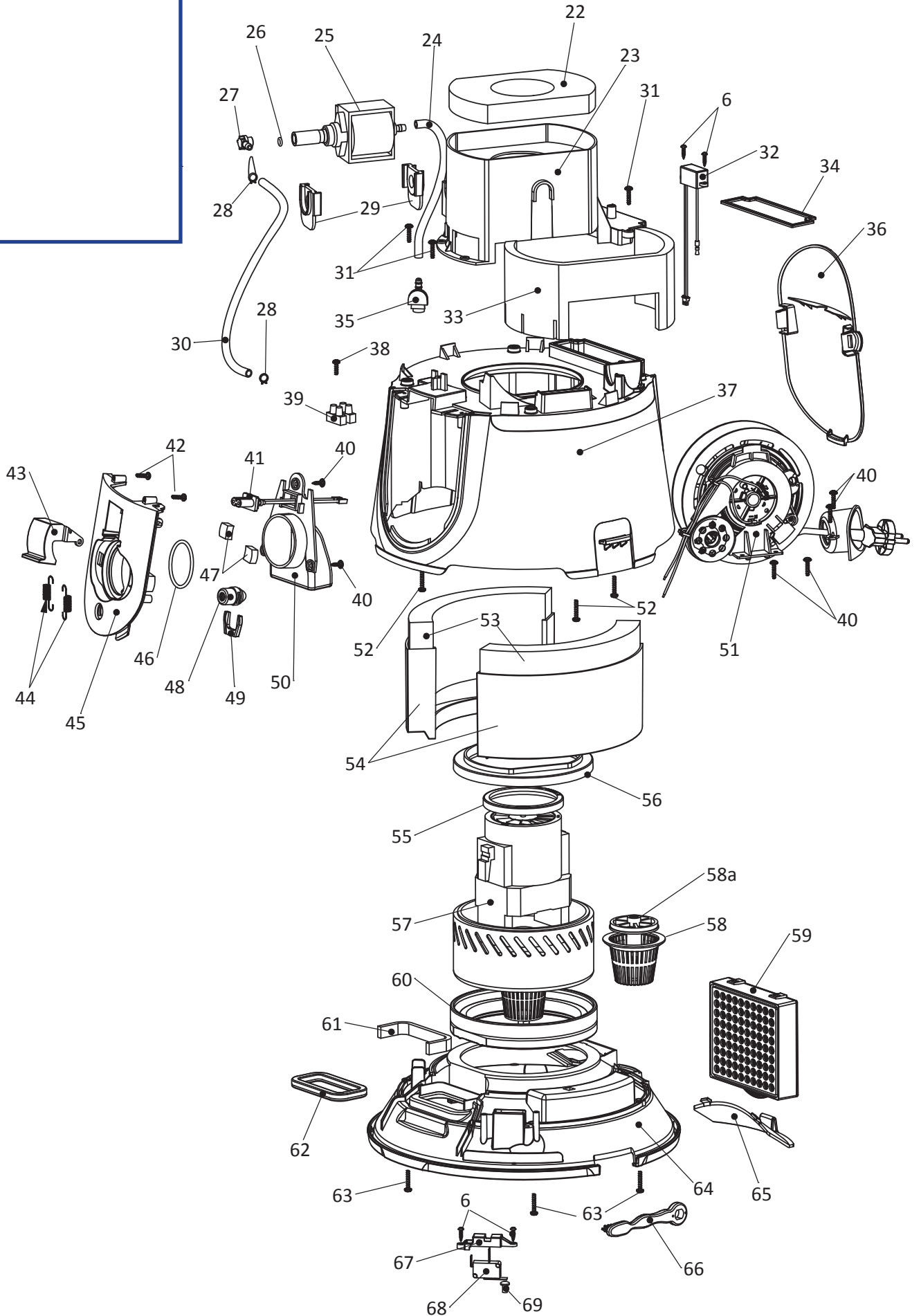
Şekil 1B - Gövde Grubu
