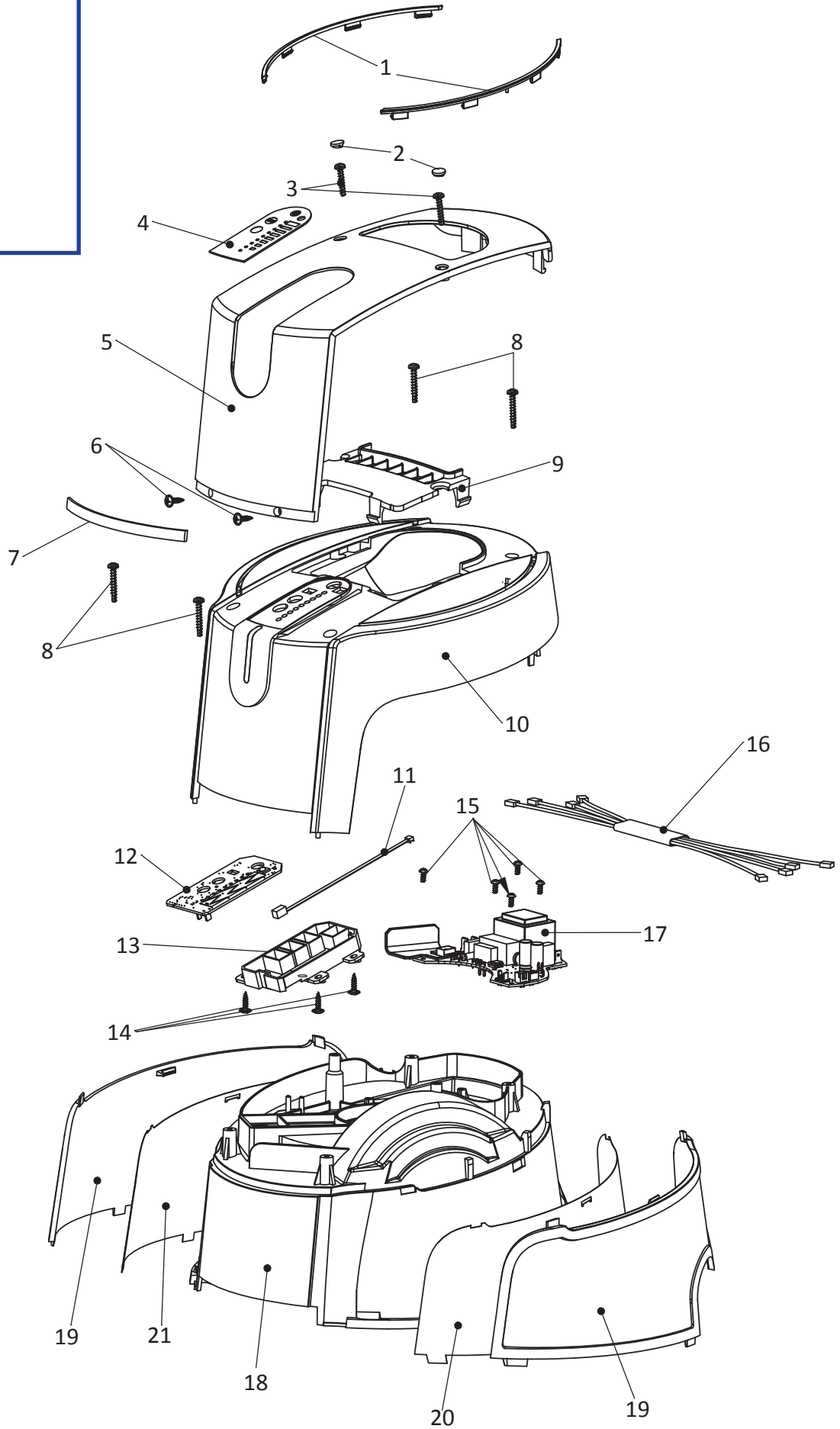
Şekil 1A - Üst Gövde Grubu
