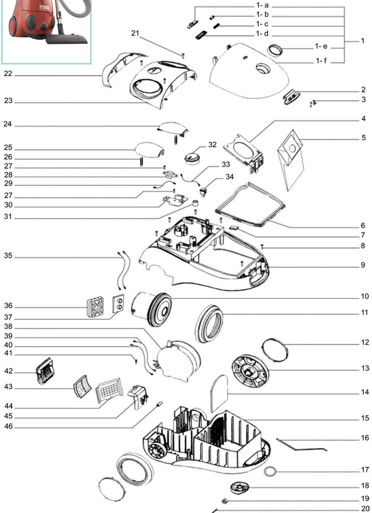
Şekil 68A - Gövde Grubu
