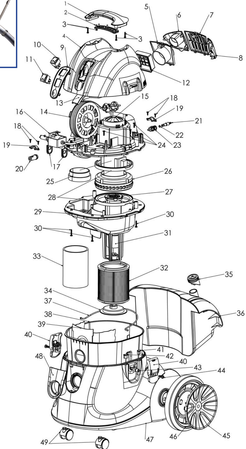
Şekil 15A - Gövde Grubu
