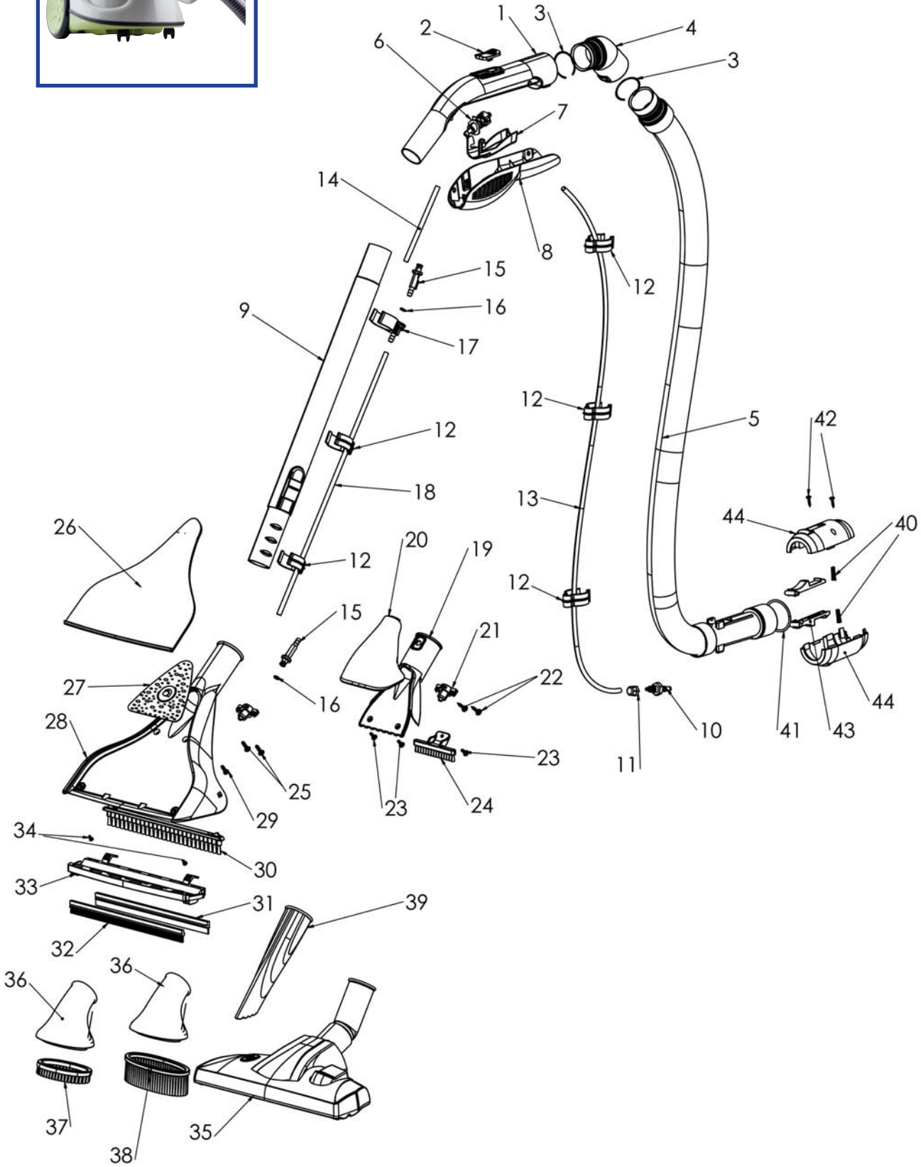
Şekil 15B - Yıkama ve Süpürme Grubu
