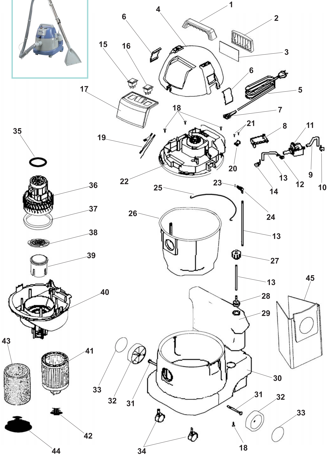
Şekil 64A - Gövde Grubu
