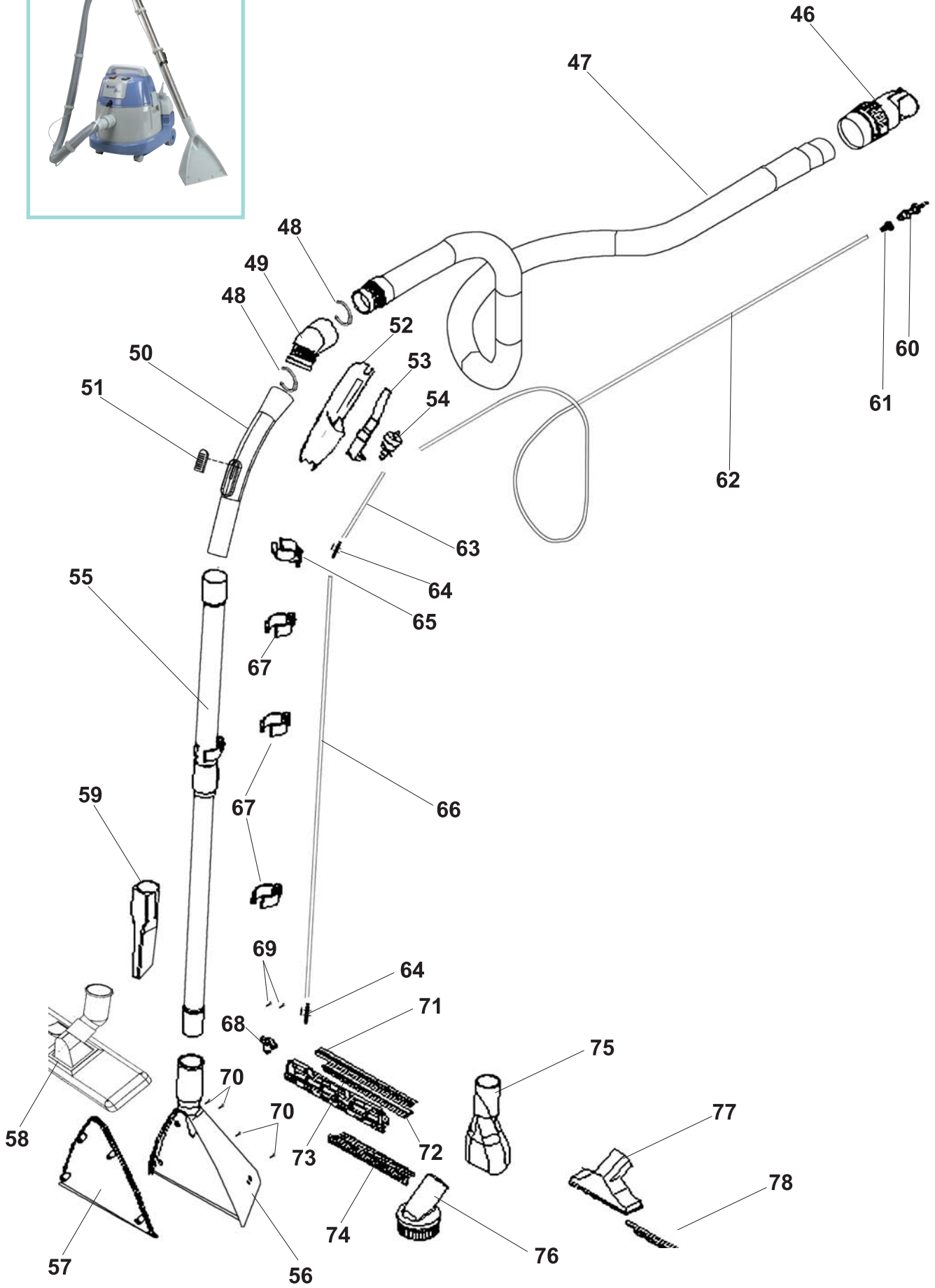
Şekil 64B - Yıkama ve Süpürme Grubu
