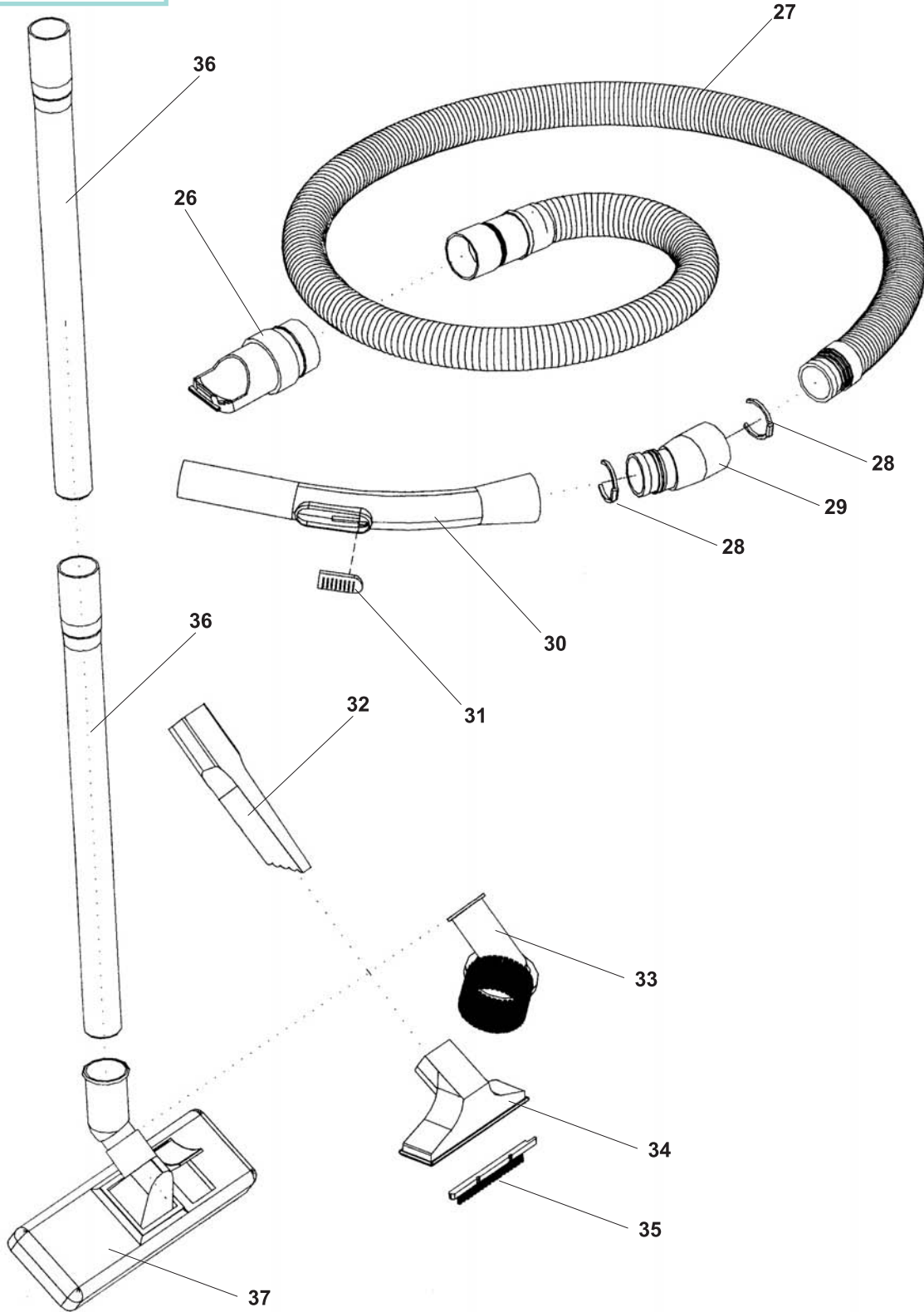
Şekil 65B - Süpürme Grubu
