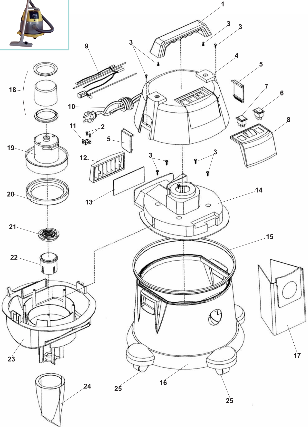
Şekil 65A - Gövde Grubu
